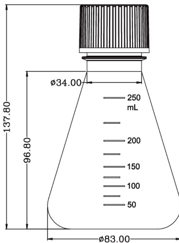
250mL Erlenmeyer Flask
